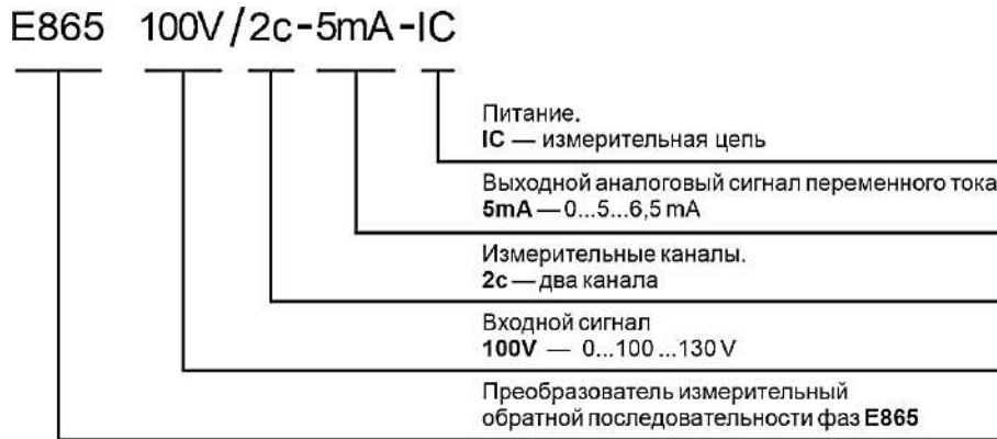
Рисунок 1 – Схема условного обозначения ИП переменного тока
