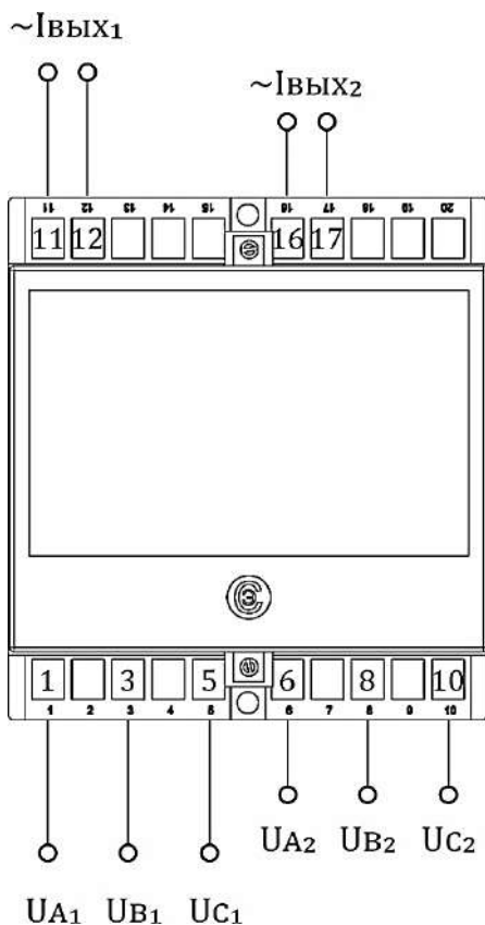
Рисунок Б.1 – Схемы электрические подключения
